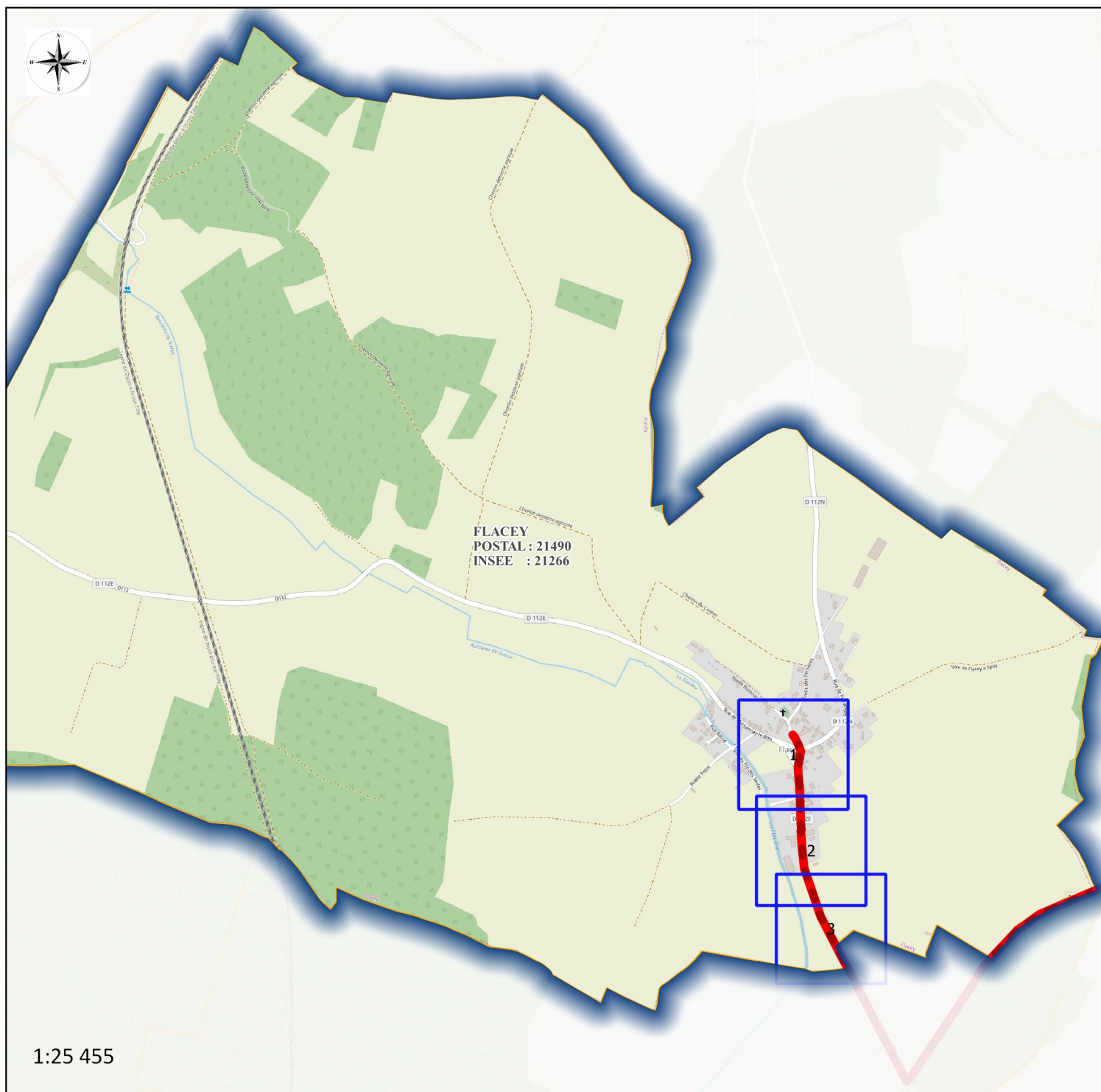
Figure 1 : vue d'ensemble du Génie Civil à réaliser sur la commune de FLACEY
