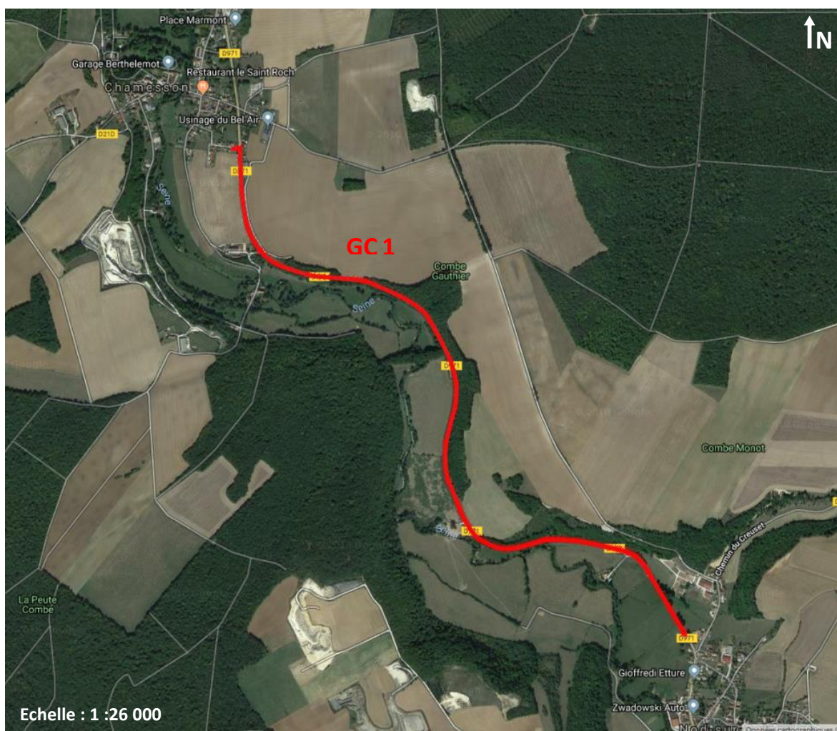
Figure 1: vue d'ensemble du Génie Civil à réaliser entre les communes de Chamesson et Nod-sur-Seine
