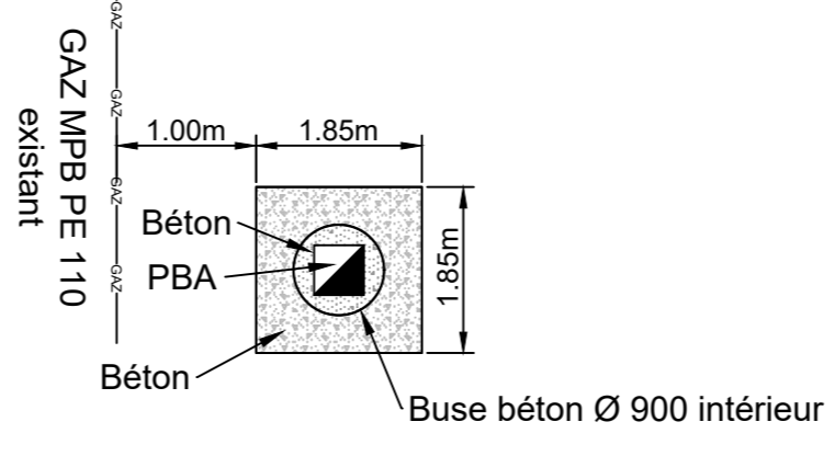
Schéma fouille pour pose PBA 2 vue de dessus
